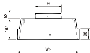
BOX-T Plenums
