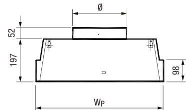
BOX-T Plénum
