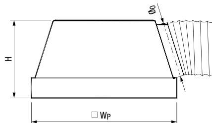
Plénum ISOBOX-R Plénum de distribution
