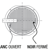
Registre de réglage Jeu de cordons pour le réglage du registre
