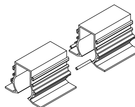
Jonction pour diffuseurs linéaires
