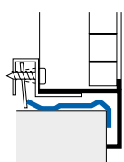
AE780 fissaggio con nottolino e controtelaio
