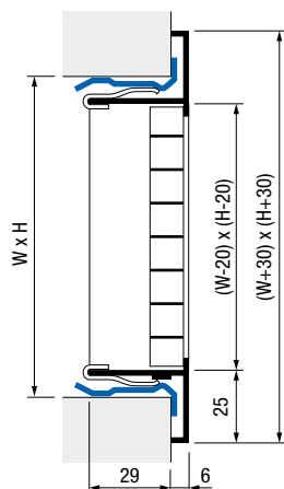
AD780 fissaggio con clips e controtelaio
