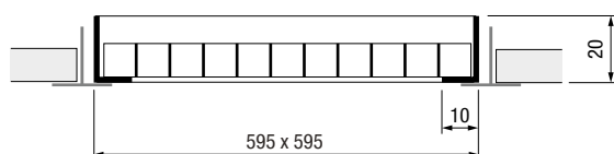
AU780 griglia per controsoffitto
