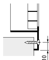
AF780 fissaggio con viti
