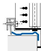
GE130 + GR001 fissaggio con nottolino e controtelaio
