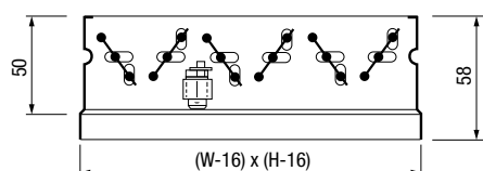
GT007 Serranda in acciaio zincato
