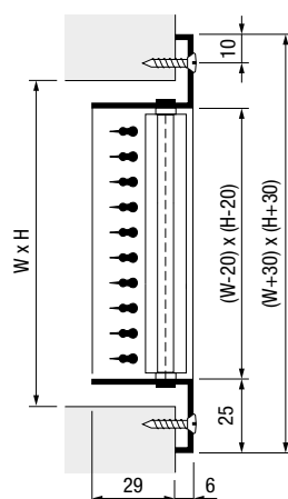
GF130 fissaggio con viti in vista
