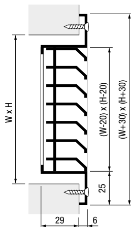
type AF350 fixation par vis
