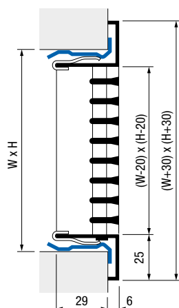
type AD360 fixation par clips et contre-cadre
