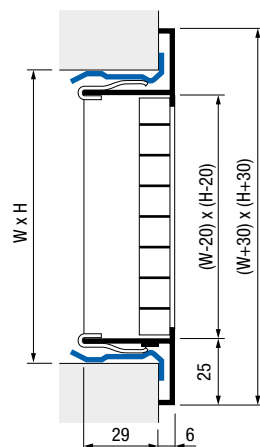
type AD780 fixation par clips et contre-cadre
