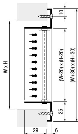
type GF130 fixation par vis
