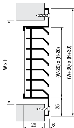
tipo AF350 fissaggio con viti
