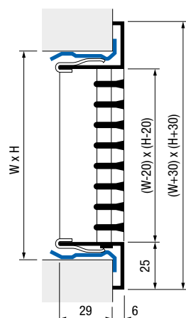
tipo AD360 fissaggio con clips e controtelaio
