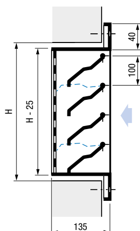
GP101S Avec grillage de 25 x 12 x 1,5 mm Soit l'ouverture W x H, corps net de la grille (W - 25) x (H - 25)
