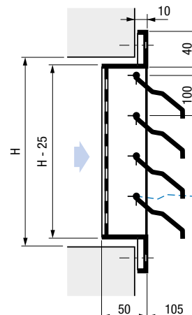
GP101D Avec grillage de 25 x 12 x 1,5 mm
