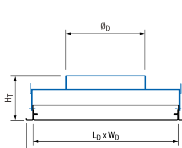
BPT-DB Plénum avec piquage sur le dessus
