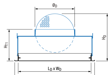
BPT/D-DB Plénum avec piquage sur le dessus et registre
