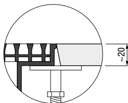
LMT-SHD1 fissaggio in appoggio al pavimento
