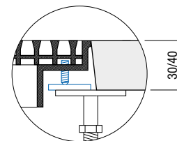
LMT-SHDA fissaggio con viti
